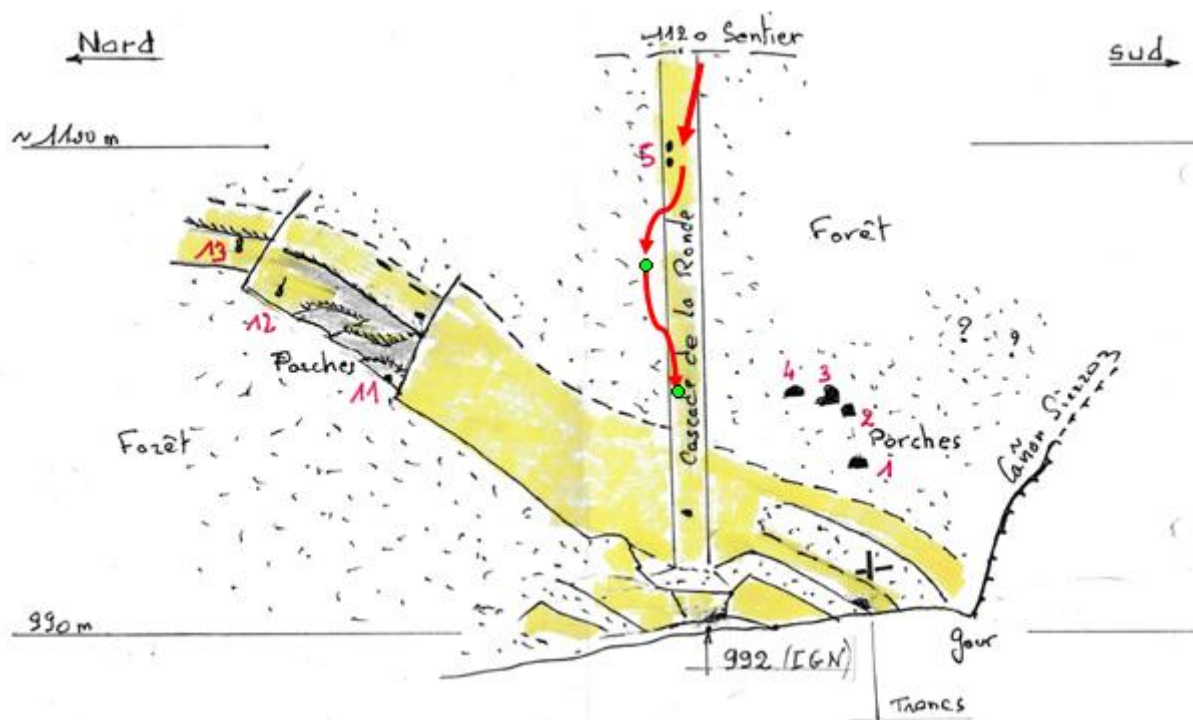
Schéma de la cascade de La Ronde vue du versant opposé. En haut, le sentier est à la cote 1120 (ligne de niveau sur la carte). En bas de la cascade, c'est la confluence Ronde/Sierroz à la cote 992 (point coté sur la carte).
