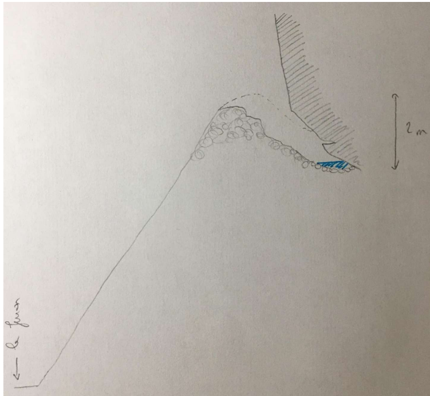
Coupe schématique de l'exsurgence Salmotrou.
